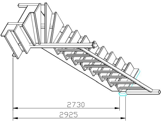
СТАНДАРТНАЯ ЛЕСТНИЦА К-001
